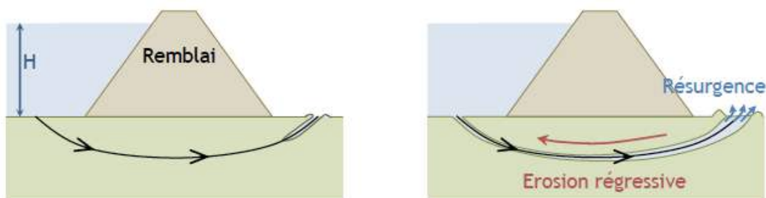
Figure 80: Illustration en deux phases du phénomène de renard en fondation (extrait de DESODT et MOLINARO (2016)).
