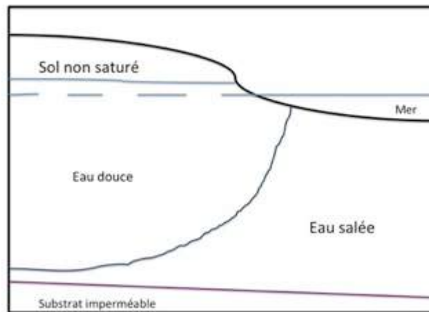
Figure 14 : Représentation schématique d'un biseau salé (extrait de http://hmf.enseeiht.fr/travaux/CD0809/bei/beiere/groupe2/node/154 )
