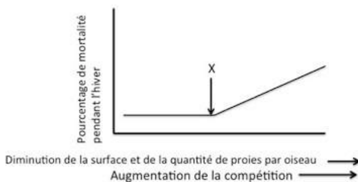
Figure 19 : L'importance de la densité dépendance dans la détermination de la réponse des populations à un changement environnemental ; forme attendue des fonctions de mortalité densité-dépendante.
