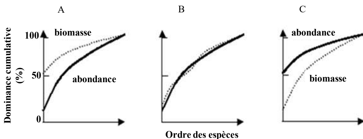
Figure 64 : Courbes de dominance k pour la biomasse et l'abondance sous trois scénarios de stress écologique selon WARWICK (1986). A = absence de stress; B = stress modéré; C = stress élevé.
