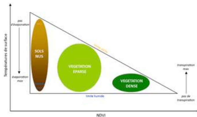
Figure 63 : Relation simplifiée entre la température de surface et l'indice de végétation (d'après LAMBIN et ERLICH, 1996).
