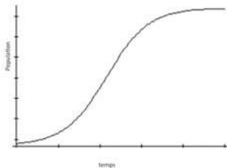
Figure 82 : Forme classique de la réponse numérique.
