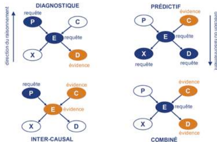
Figure 84 : Types de raisonnements dans un Réseau Bayésien (d'après KORB et NICHOLSON, 2004).
