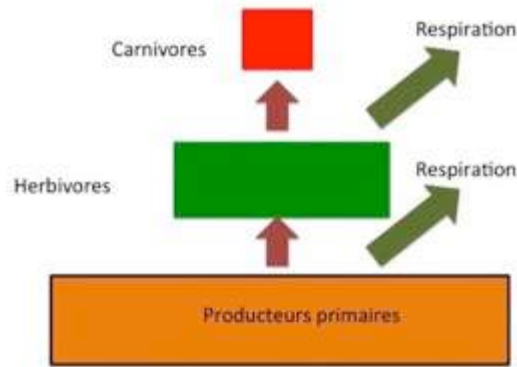
Figure 31 : Exemple simplifié de chaînes de producteurs et de consommateurs
