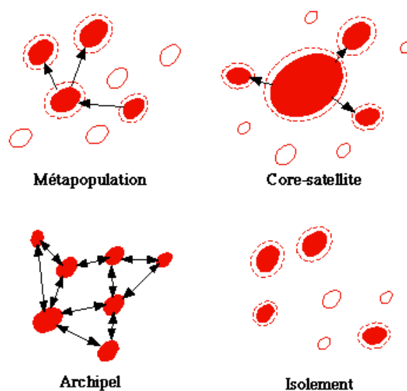
Figure 67 : Les différents types de distribution des populations.
