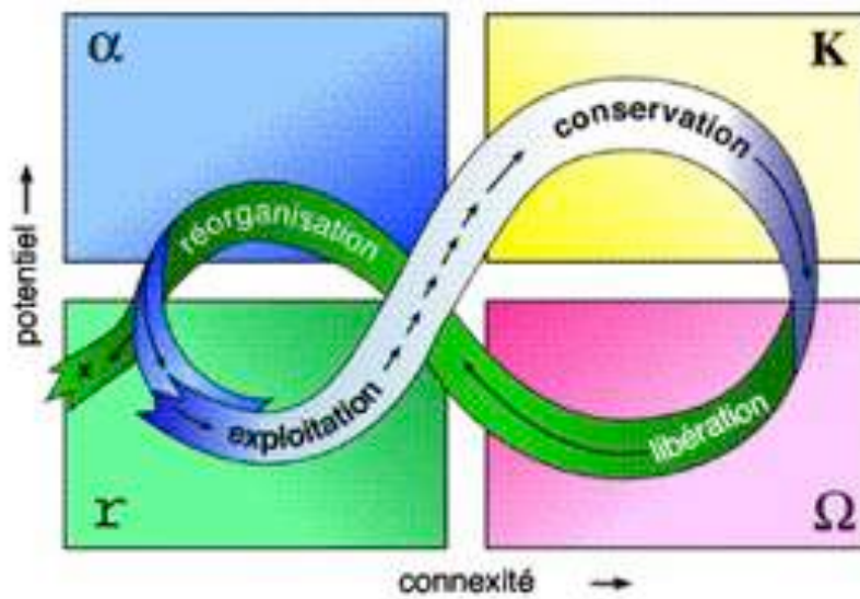
Figure 35 : Représentation du cycle adaptatif.
