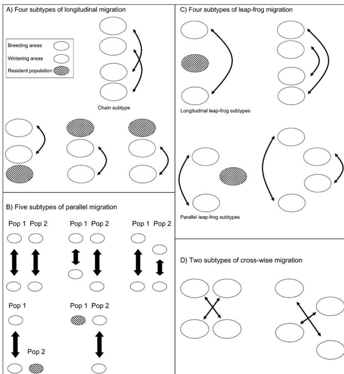
Figure 30 : Les types théoriques de systèmes de migration de Salomonsen conduisant à une forte connectivité : (A) migration longitudinale, (B) migration parallèle, (C) migration à saute-mouton et (D) migration croisée. La légende est dans le panneau A. Modifié de SALOMONSEN (1955) par BOULET et NORRIS (2006).
