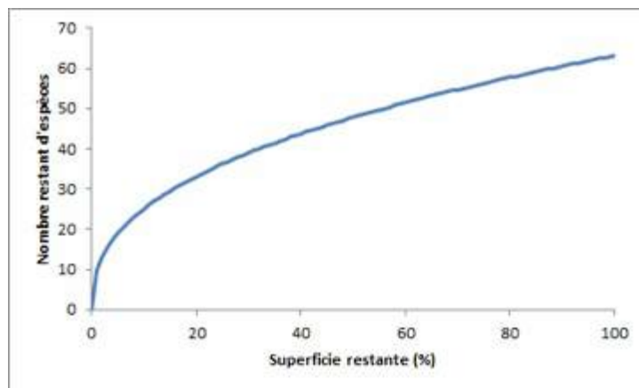
Figure 33 : Courbe aire – espèces.
