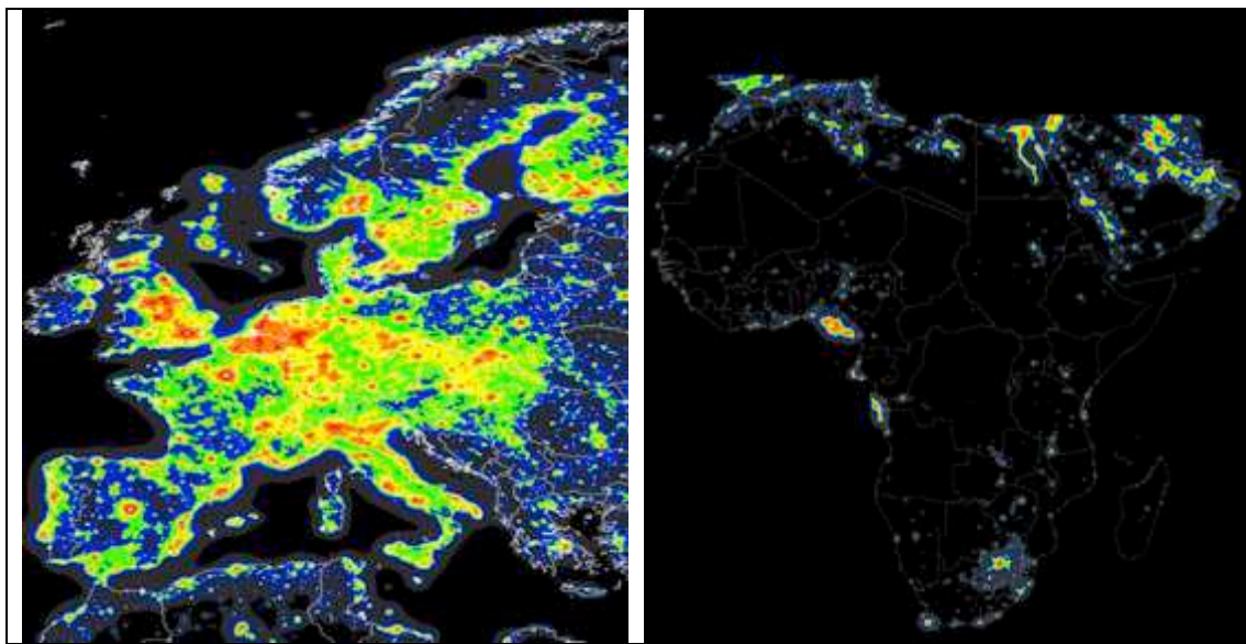
Figure 76 : La pollution lumineuse en Europe, à gauche, et en Afrique, à droite.
