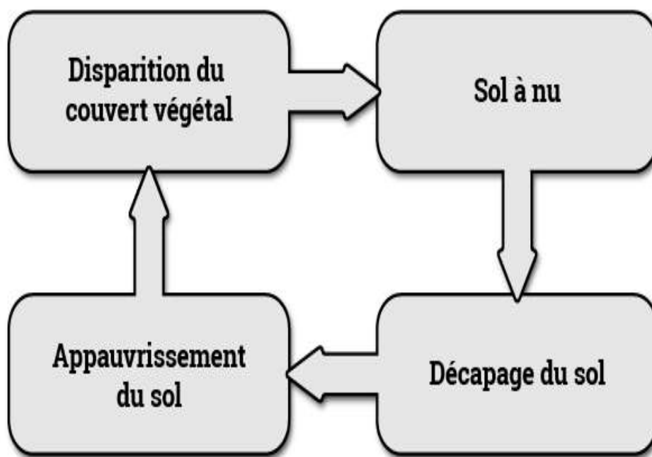
Figure 85 : principe de la rhexistasy.
