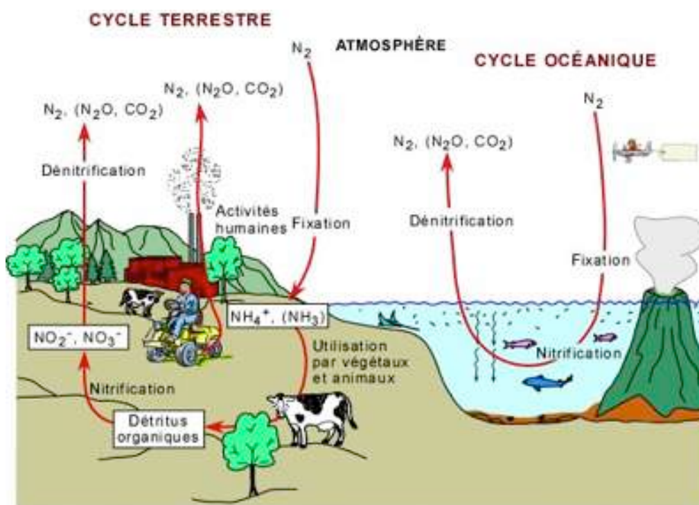
Figure 39 : Représentation schématique du cycle de l'azote.
