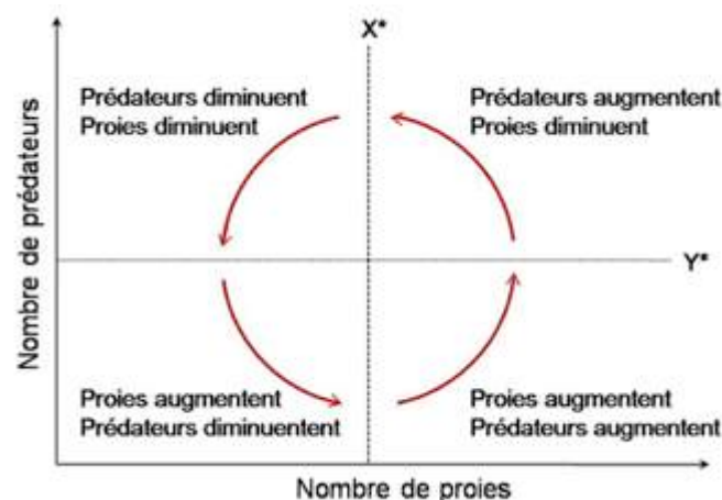
Figure 48 : Espaces des phases du modèle de Lotka-Volterra et évolution de l'abondance des proies et des prédateurs.
