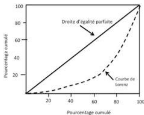
Figure 34 : Exemple de courbe de Lorenz.
