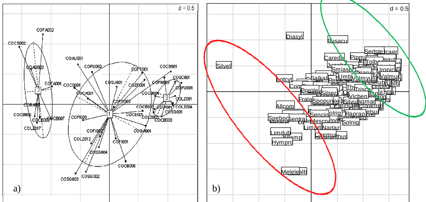
Figure 2 : Analyse NMDS réalisée sur les données floristiques de 39 îles corses, sans les espèces peu communes (a : représentation des îles ; b : représentation des espèces).
