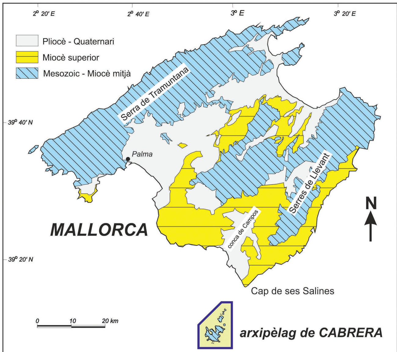
Figura 1 Localització i mapa geològic simplificat.
