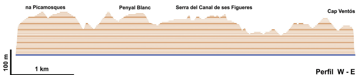
Figura 6 Perfil de l'illa de Cabrera projectat des del sud sobre un pla imaginari W-E (exageració vertical: x4).
