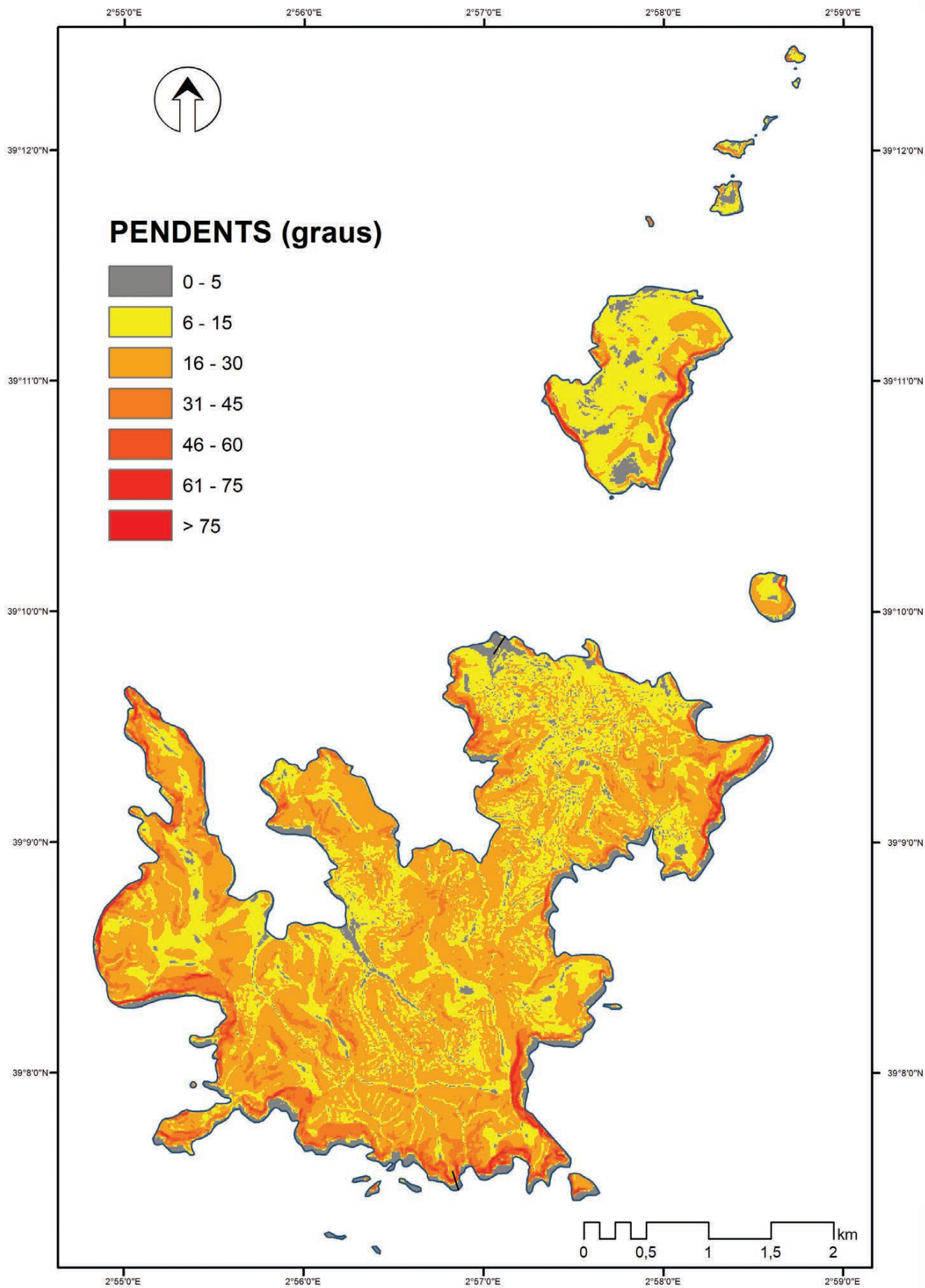
Figura 7 Mapa de pendents de Cabrera confeccionat a partir del núvol de punts LIDAR 2014 de l'IGN.
